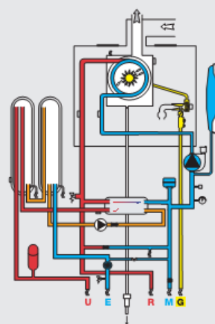
Zamknięta komora spalania - model FF
