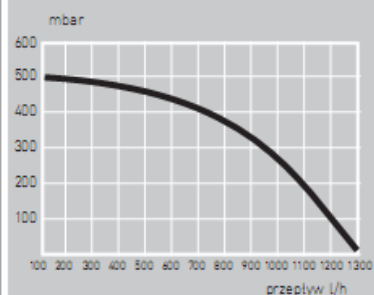
Wykres oporów przepływu przez kocioł
