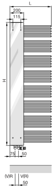
Widok z przodu: rury w prawą stronę
