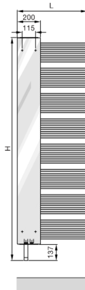
Widok z przodu: wersja elektryczna – rury w prawą stronę
