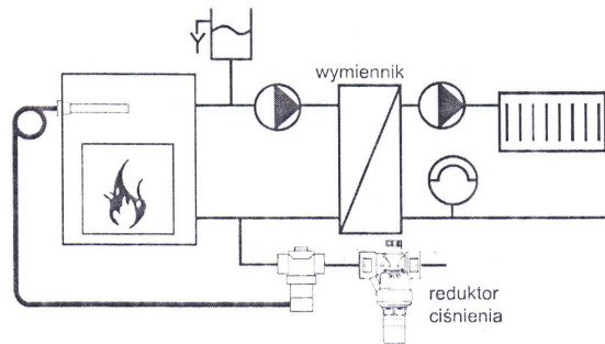
rys.3 Instalacja z naczyniem wzbiorczym systemu otwartego
