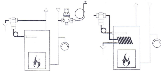
rys.3 Instalacja z naczyniem wzbiorczym systemu otwartego
