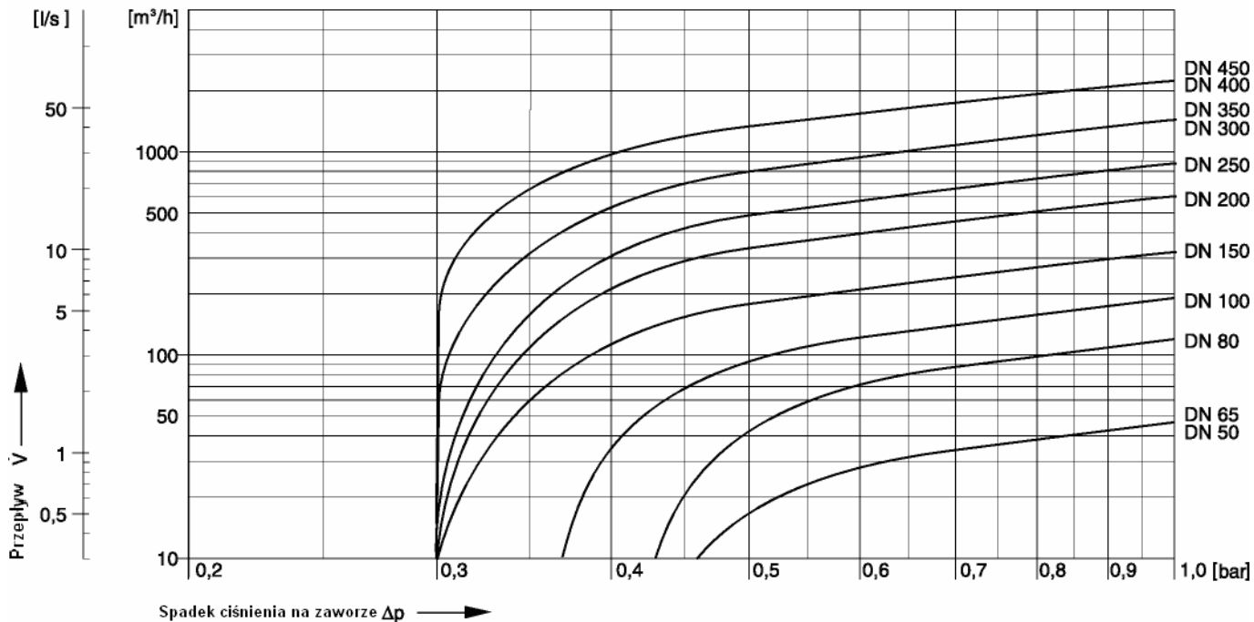
WYKRES PRZEPLYWU
