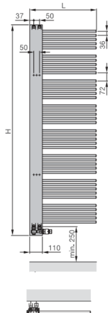
Widok z przodu: rury w prawą stronę
