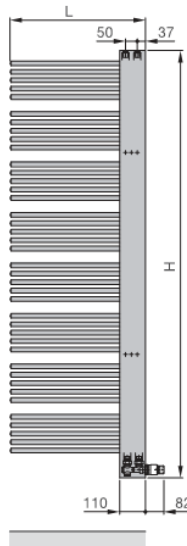
Widok z przodu: rury w lewą stronę
