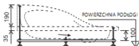
BASE Zestaw regulowanych nóg, służących do ustawienia brodzików z siedziskiem TAURUS lub TOSCA
