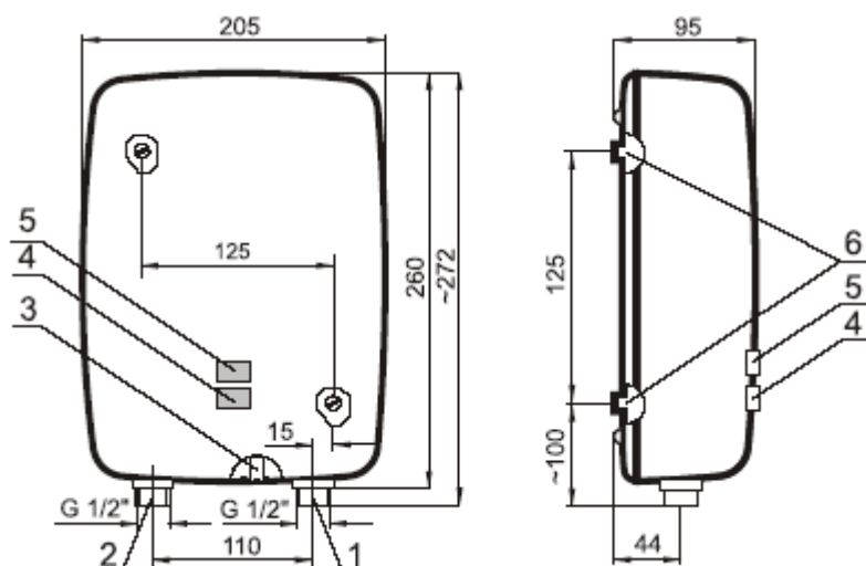
Rys. 1 Widok zewnętrzny i wymiary ogrzewacza - wersja nadumywalkowa
