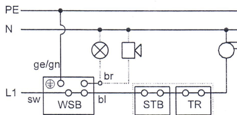
Schemat elektryczny podłączenia:
