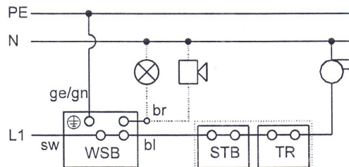
Schemat elektryczny podłączenia:
