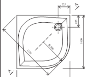
ELIPSO 100 LA, EX, PAN
