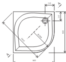
ELIPSO 90 LA, EX, PAN
